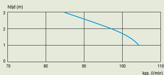
Tryckhöjd och horisontell pumpning
