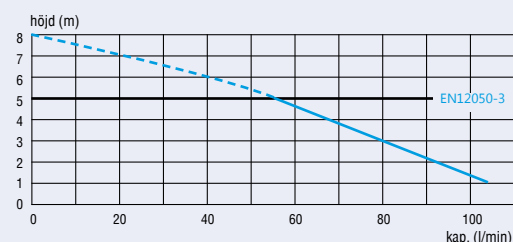
Tryckhöjd och horisontell pumpning
