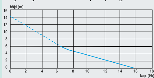
Tryckhöjd och horisontell pumpning
