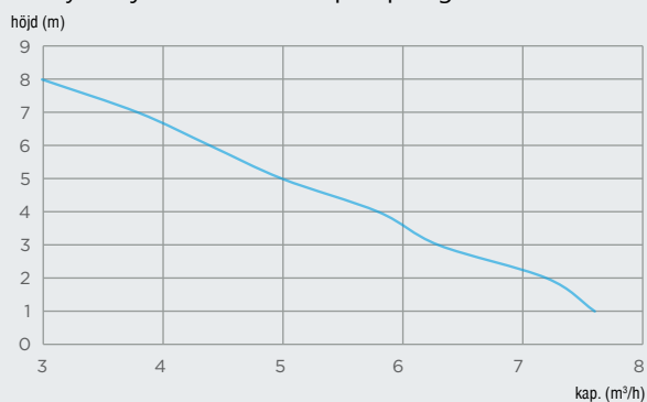
Tryckhöjd och horisontell pumpning
