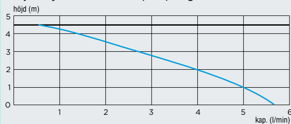
Tryckhöjd och horisontell pumpning
