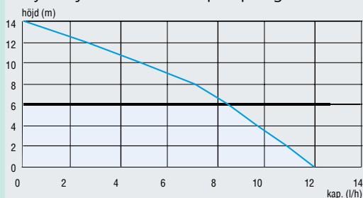
Tryckhöjd och horisontell pumpning
