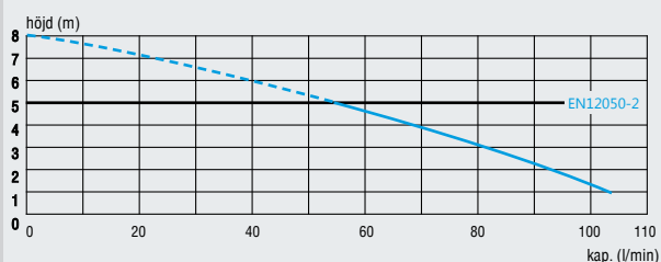
Tryckhöjd och horisontell pumpning
