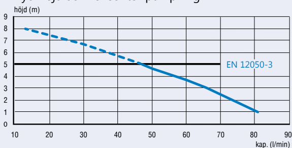
Tryckhöjd och horisontell pumpning
